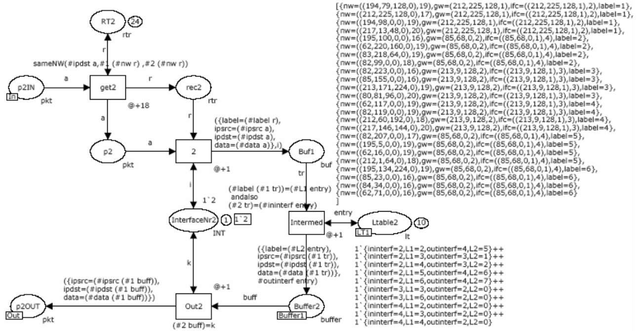
Рис. 5. Модель LER порта MPLS маршрутизатора
